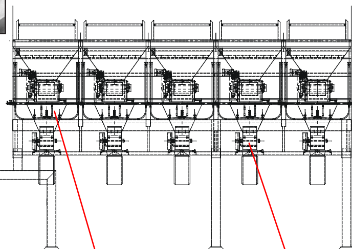
Trémie de réception/d'alimentation
