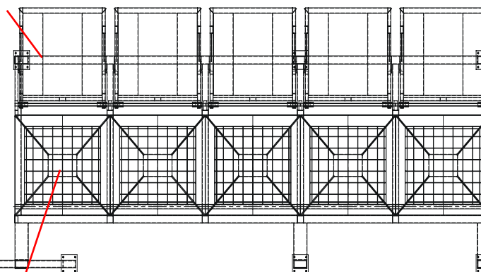
Trémie de réception/d'alimentation
